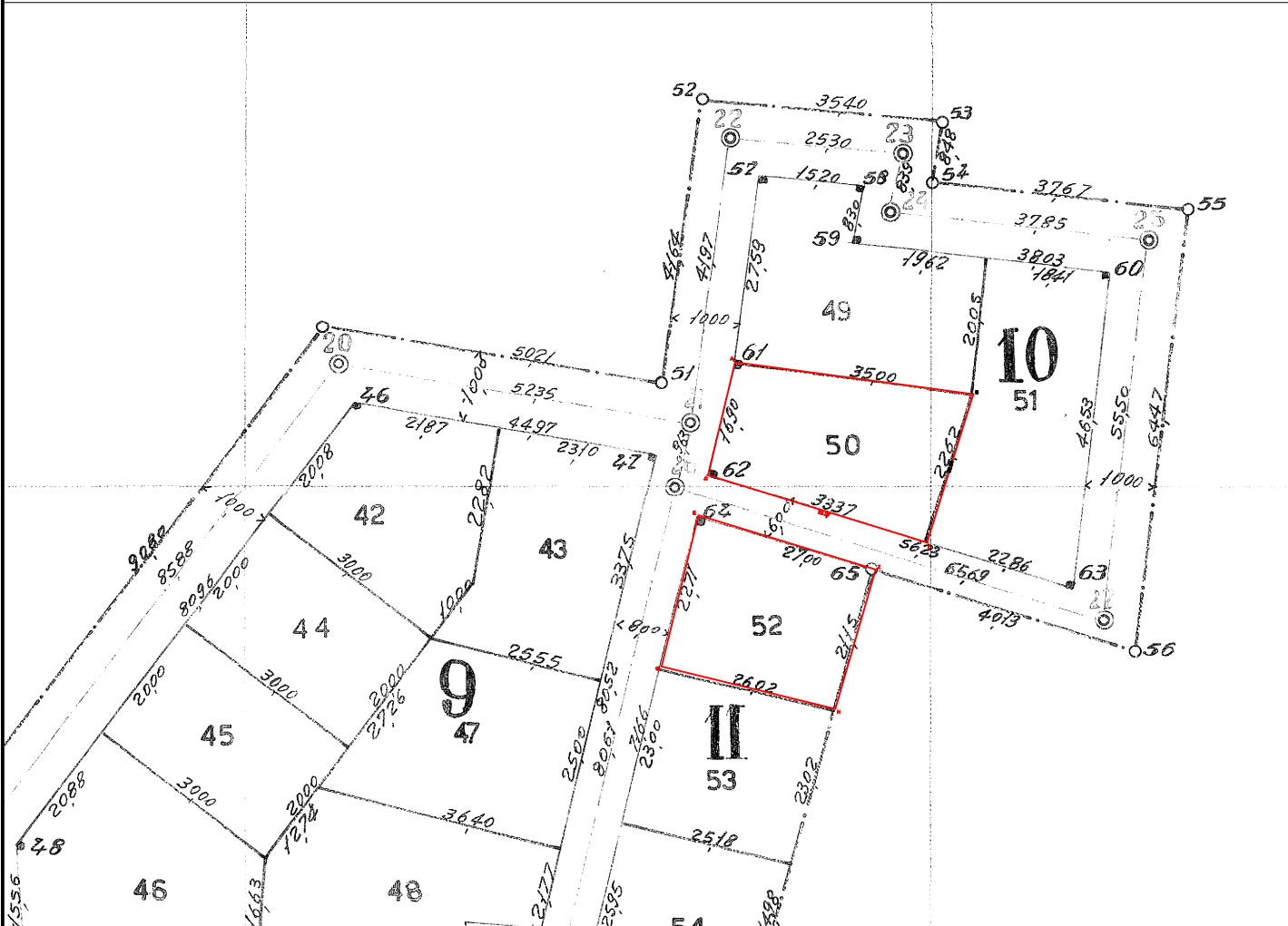
ΠΙΝΑΚΑΣ ΣΥΝΤΕΤΑΓΜΕΝΩΝ ΚΟΡΥΦΩΝ ΟΙΚΟΠΕΔΟΥ ΥΠ' ΑΡ. 50 ΜΕ ΣΤΟΙΧΕΙΑ Α-Β-Γ-Δ-Α (ΕΓΣΑ 87)
