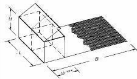
Σχήμα 4: Συρματοκιβώτια με προέκταση συρματοπλέγματος τύπου
