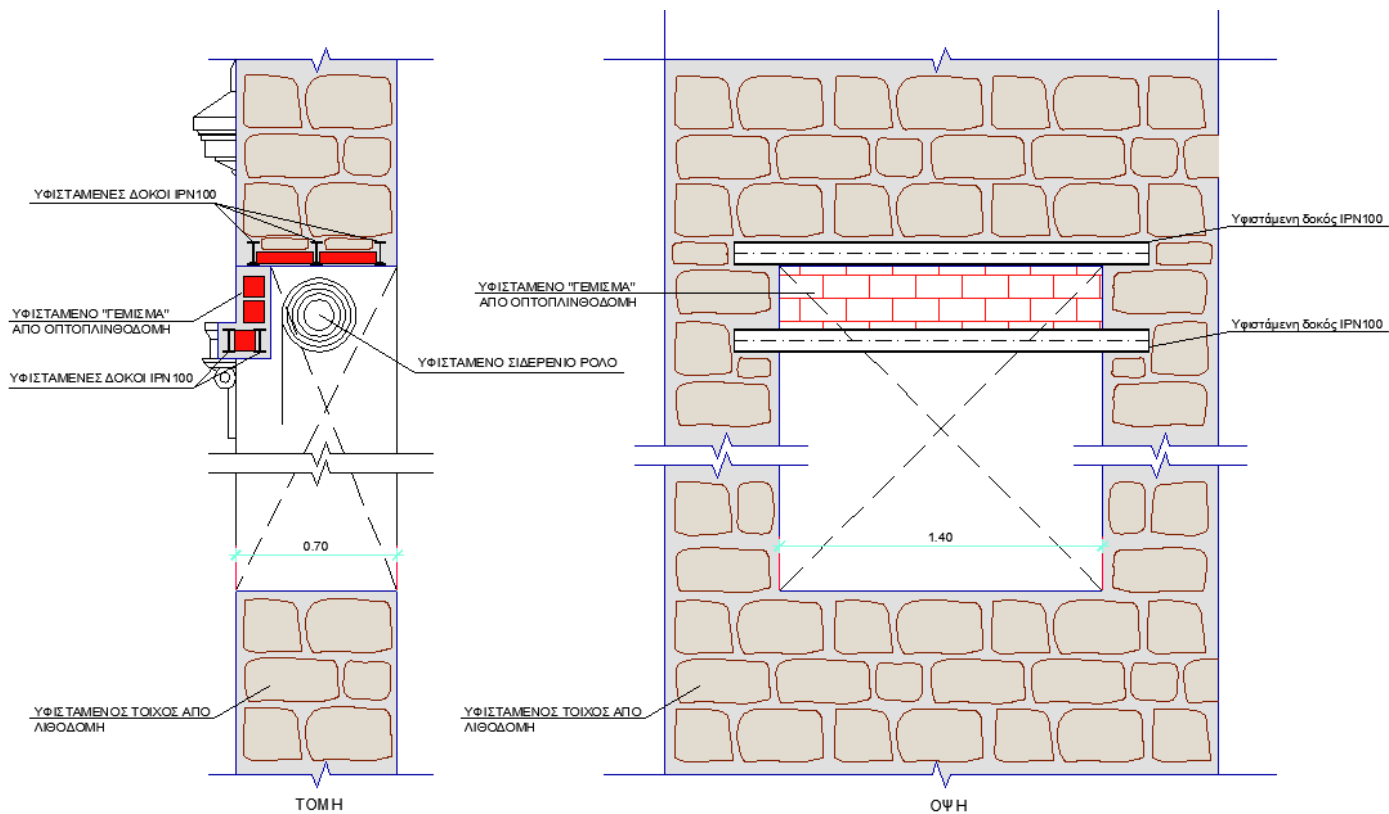
ΠΕΡΙΠΤΩΣΗ Β ΤΥΠΙΚΗ ΛΕΠΤΟΜΕΡΕΙΑ ΥΦΙΣΤΑΜΕΝΗΣ ΚΑΤΑΣΤΑΣΗΣ ΑΝΩΦΛΙΩΝ (ΥΠΕΡΘΥΡΑ) ΠΑΡΑΘΥΡΩΝ ΤΟΙΧΟΥ ΑΠΟ ΛΙΘΟΔΟΜΗ ΠΑΡΑΘΥΡΑ 3ου & 4ου ΟΡΟΦΟΥ ΔΥΤΙΚΗΣ & ΝΟΤΙΑΣ ΟΨΗΣ
